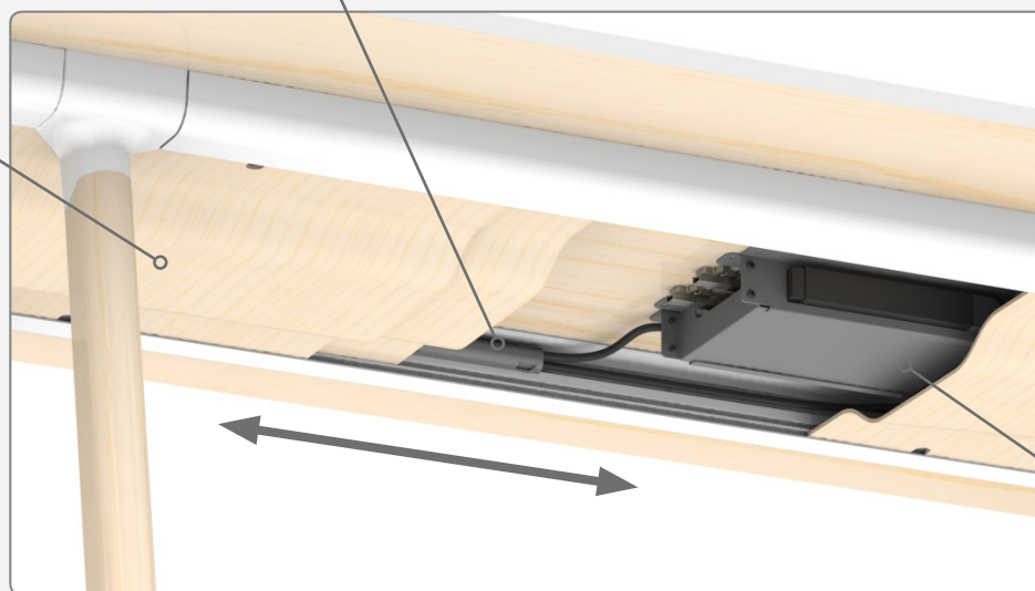
Cable clip
